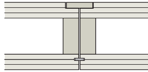
Variante 35 Languette 9 mm x 30 mm Battue standard 23/51 mm alternative 23/51 mm CLT BOX – DALLE, Hauteur : de 220 mm à 480 mm CLT BOX – DALLE FS, Hauteur : de 260 mm à 490 mm
