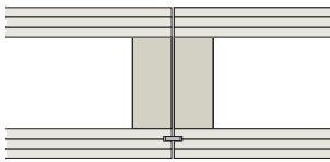
Variante 32 Languette 9 mm x 30 mm CLT BOX – DALLE, Hauteur : de 220–480 mm CLT BOX – DALLE FS, Hauteur : de 260 à 490 mm
