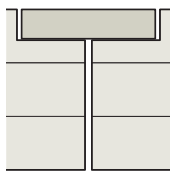
Variante 13 Battue standard 23/51 mm alternative 28/51 mm Épaisseur : de 60 à 280 mm
