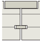
Variante 15 Languette 9 mm x 30 mm Battue standard 23/51 mm alternative 28/51 mm Épaisseur : de 100mm à 280 mm
