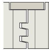
Variante 4 Double rainure et languette 2cm Battue standard 23/51 mm alternative 28/51 mm Battue spéciale max. 30/68 mm
