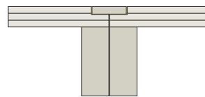
Variante 43 Battue standard 23/51 mm alternative 28/51 mm Hauteur : de 160 mm à 490 mm
