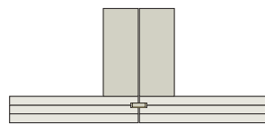
Variante 42 Languette 9 mm x 30 mm Épaisseur : de 160 mm à 490 mm
