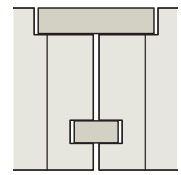
Variante 5 Languette 19 mm x 38 mm Battue standard 23/51 mm alternative 28/51 mm Battue spéciale max. 30/68 mm
