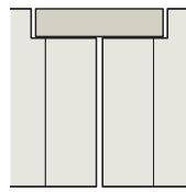
Variante 3 Battue standard 23/51 mm alternative 28/51 mm Battue spéciale max. 30/68 mm
