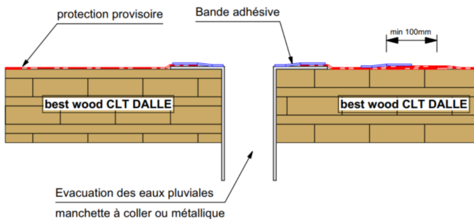
Figure 13 : Jonction de la protection temporaire avec une évacuation pluviale
