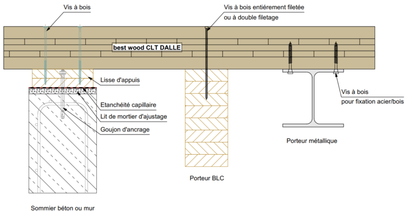
Figure 3 : Plancher – Appuis usuels sur support béton, bois ou métallique
