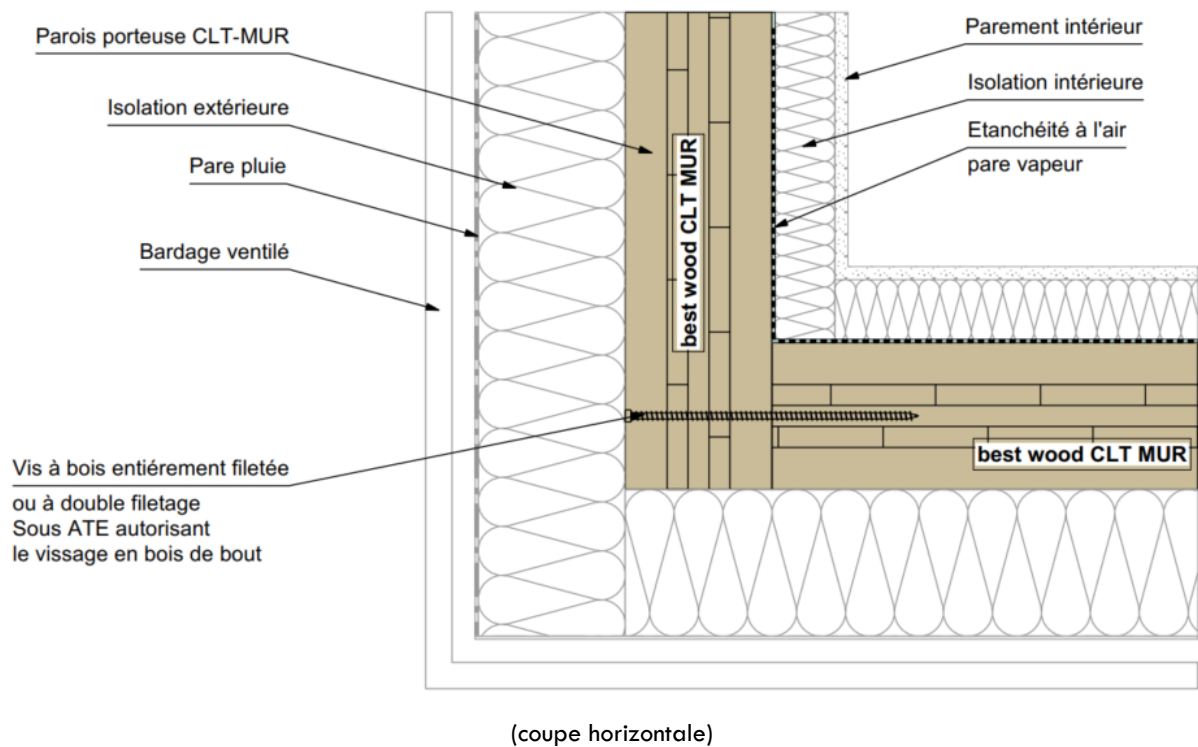
Figure 6 : Mur – Exemples d'assemblage des panneaux best wood CLT entre eux – Angle sortant de murs extérieurs
