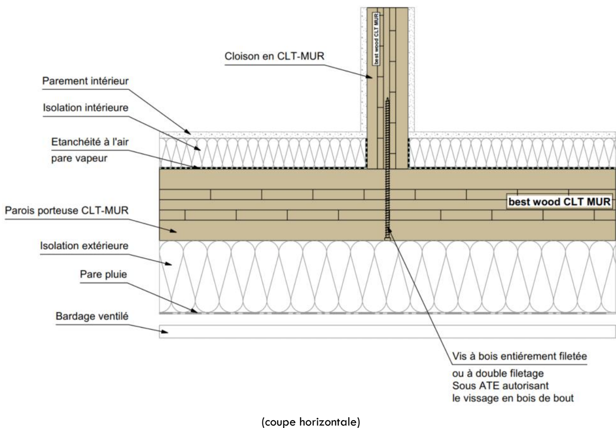
Figure 7 : Mur – Exemples d'assemblage des panneaux best wood CLT entre eux – Liaison mur extérieur / mur de refend
