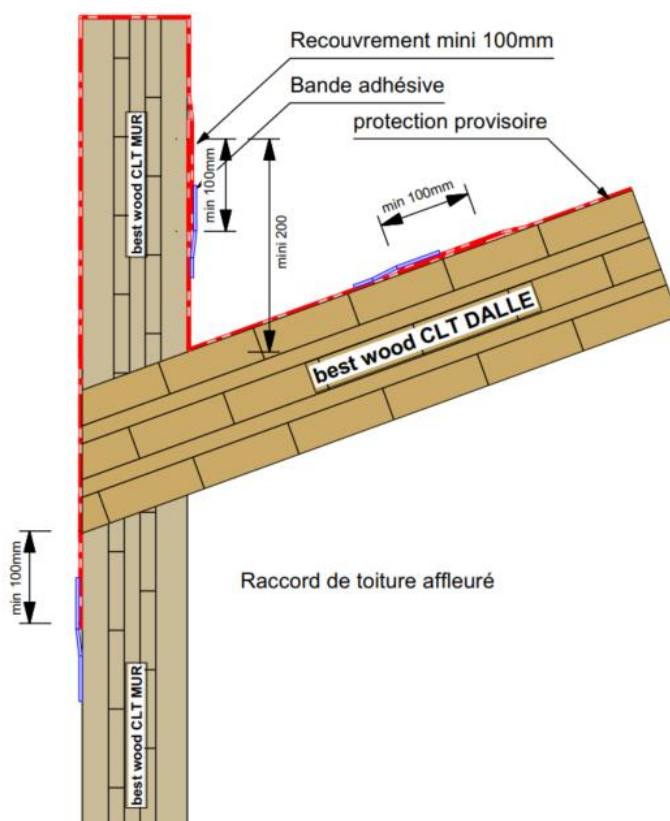
Figure 15 : Gestion d'un relief par protection temporaire
