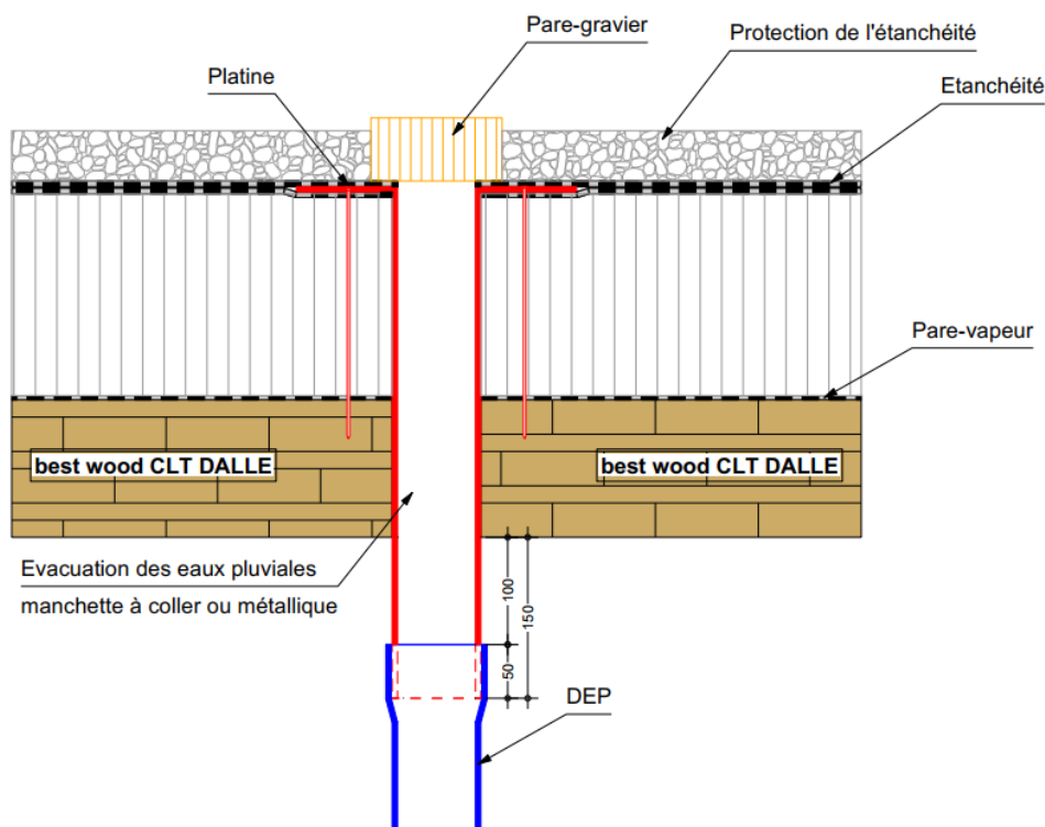
Figure 28 : Toiture chaude isolée inaccessible – Entrée d'eaux pluviales avec pare-gravier
