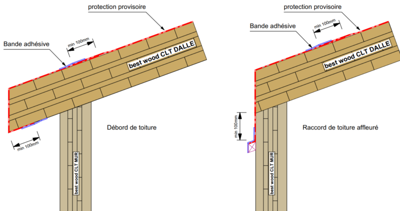
Figure 12 : Gestion de la protection temporaire en bas de pente
