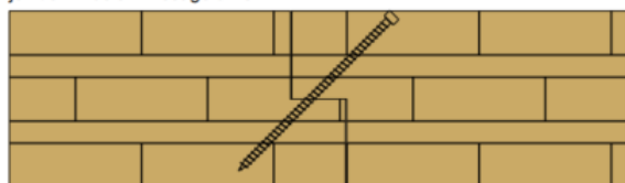
Figure 1 : Jonction des panneaux best wood CLT entre eux – Mur
