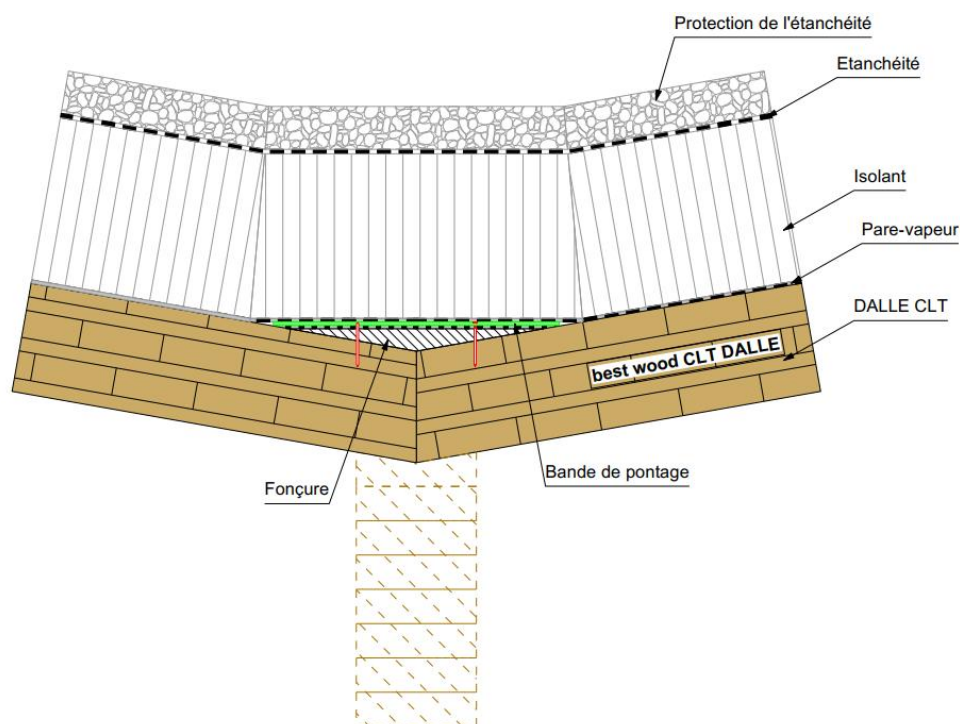
Figure 25 : Toiture chaude isolée inaccessible – Noue avec fondure
