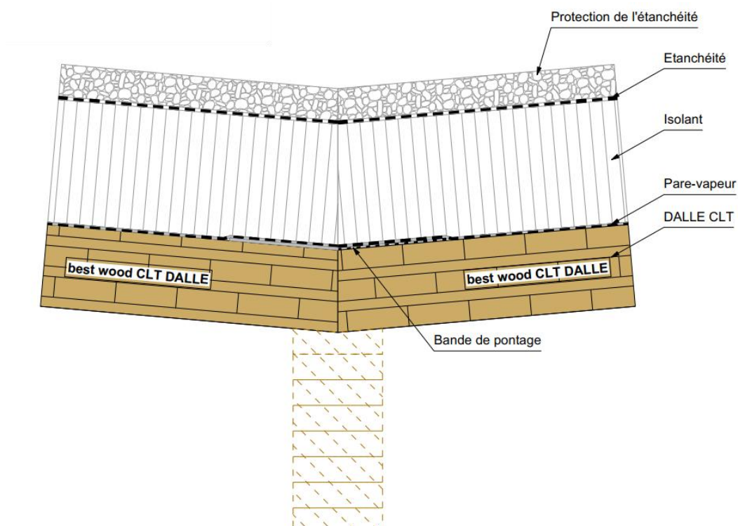
Figure 24 : Toiture chaude isolée inaccessible – Noue
