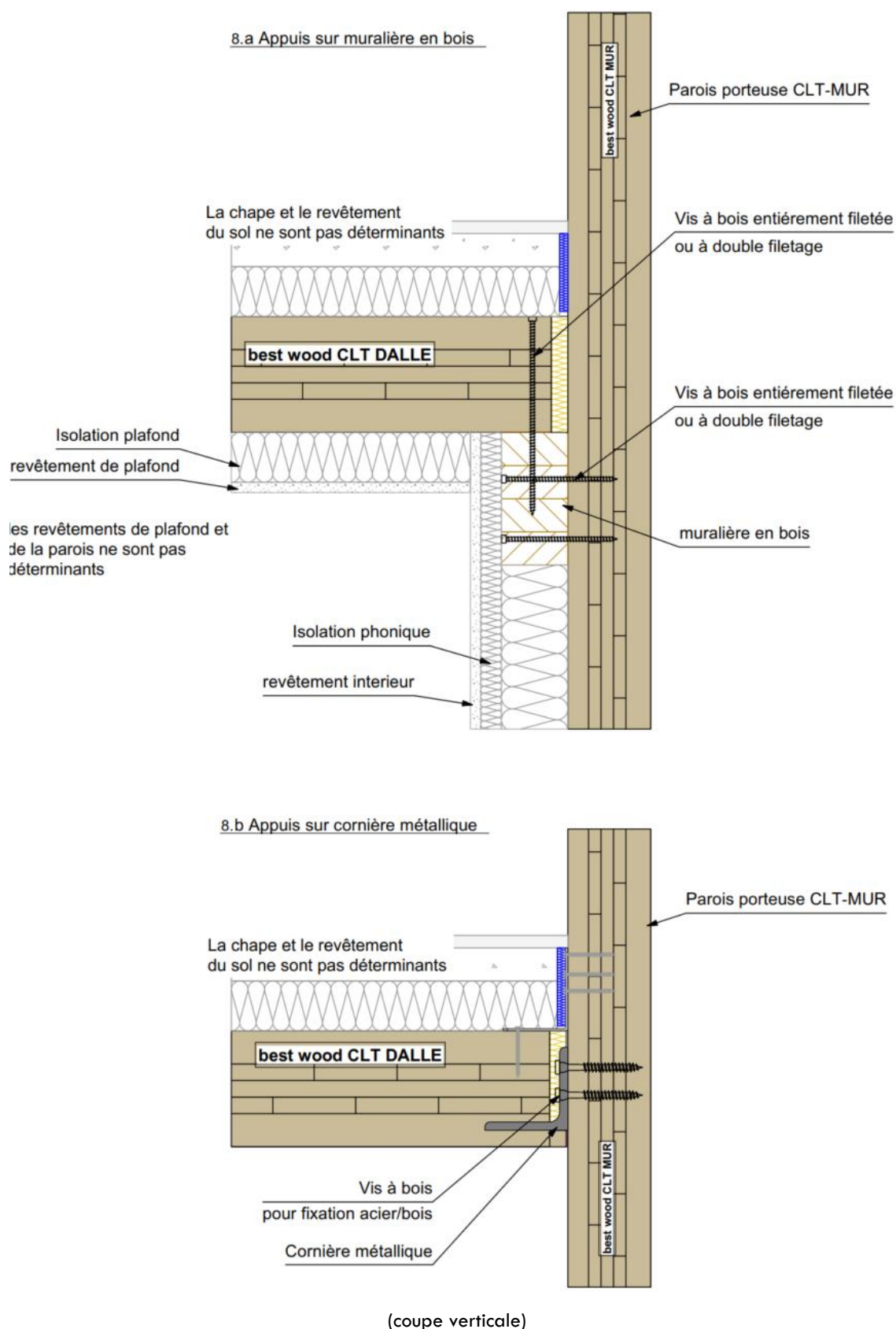
Figure 8 : Mur et Plancher – Exemples d'appuis de plancher sur un mur (intérieur ou extérieur) filant
