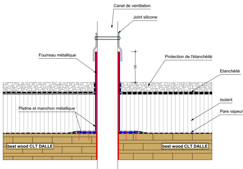
Figure 29 : Toiture chaude isolée inaccessible – Traversée de conduit de ventilation
