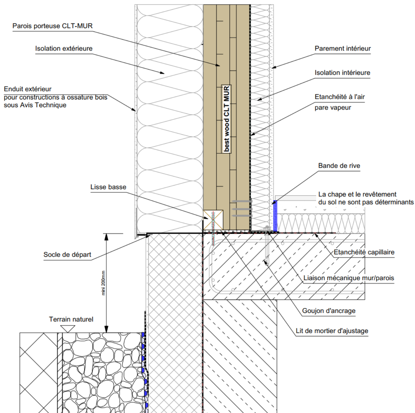
Figure 5 : Mur – Exemple d'appui de mur sur support béton avec ETICS (enduit sur ITE)
