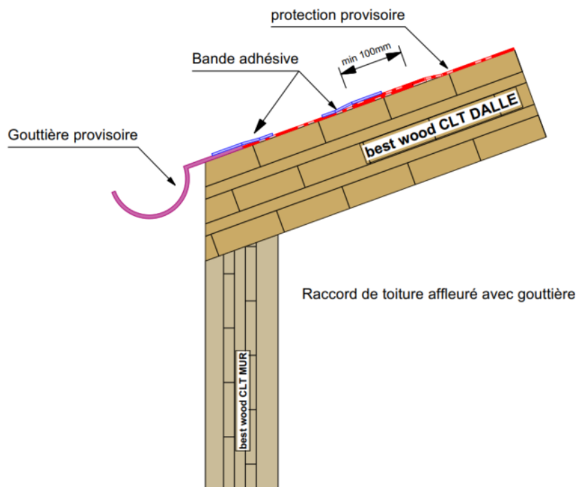
Figure 14 : Mise en œuvre d'une gouttière en bas de pente de protection temporaire
