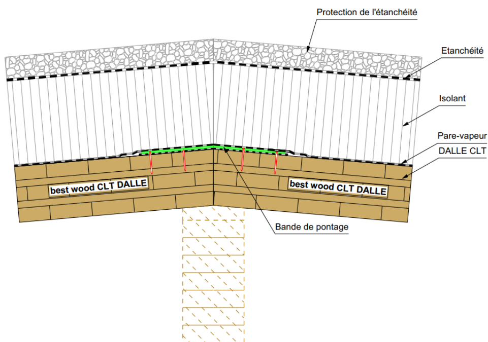
Figure 26 : Toiture chaude isolée inaccessible – Faîtage
