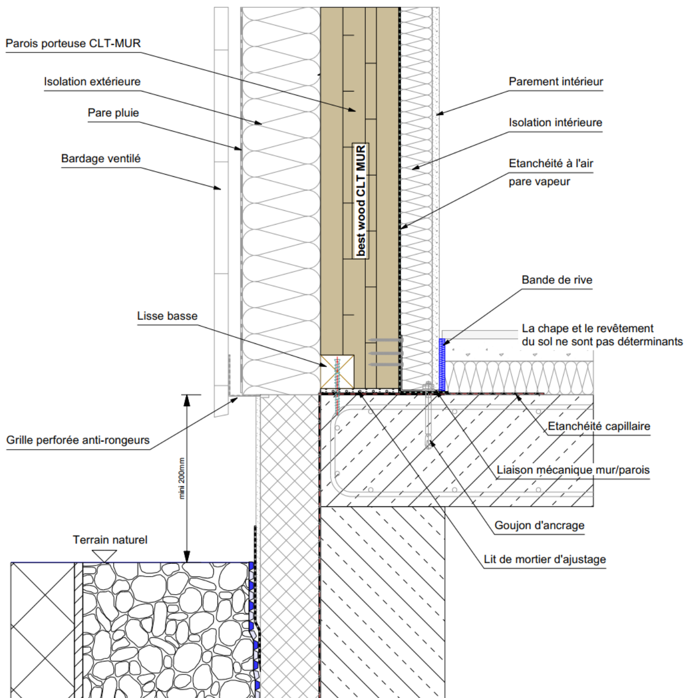
Figure 4 : Mur – Exemple d'appui de mur sur support béton avec bardage à lame d'air ventilée
