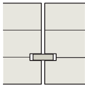
Variante 12 9 x 30 mm Fremdfeder Dicke: 60–280 mm
