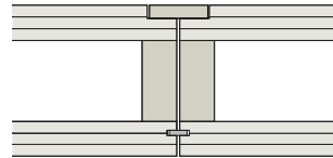
Variante 35 9 x 30 mm Fremdfeder Standardausfaltung 23/51 mm alternativ 28/51 mm CLT BOX – DECKE, Höhe: 220–480 mm CLT BOX – DECKE FS, Höhe: 260–490 mm
