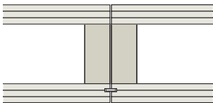
Variante 32 9 x 30 mm Fremdfeder CLT BOX – DECKE, Höhe: 220–480 mm CLT BOX – DECKE FS, Höhe: 260–490 mm
