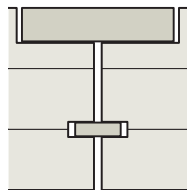
Variante 15 9 x 30 mm Fremdfeder Standardausfaltung 23/51 mm Dicke: 100–280 mm
