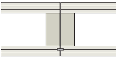
Variante 32 9 x 30 mm Fremdfeder Höhe: 260–480 mm
