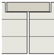
Variante 13 Standardausfaltung 23/51 mm Dicke: 60–280 mm
