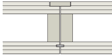
Variante 35 9 x 30 mm Fremdfeder Standardausfaltung 23/51 mm Höhe: 260–480 mm
