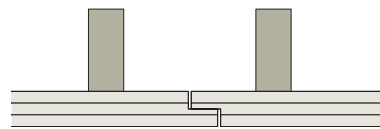
Variante 26 Stufenfalz (halbe Dicke/50 mm) Gesamthöhe: 200–480 mm
