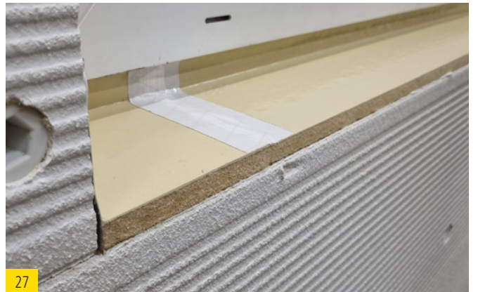
best wood KLEBEBAND gut festdrücken - gleiche Vorgehensweise an beiden Stößen.
