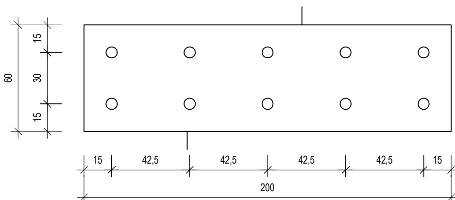
Plattenlänge 2000 mm
