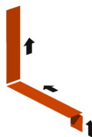
Verlauf des Fugendichtbandes um die Fensterbank und zum Fenster.
