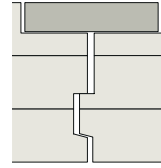
Variante 14 10 mm Nut und Feder Standardausfaltung 23/51 mm Dicke: 80–280 mm Sonderausfaltung ab 80 mm max. 27/59 mm ab 90 mm max. 35/59 mm
