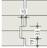
Variante 11 10 mm Nut und Feder Dicke 80–280 mm
