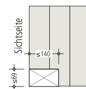
Variante 18 Falz Schwelle
