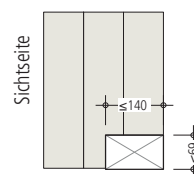
Variante 17 Falz Schwelle
