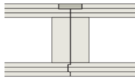
Variante 34 10 mm Nut und Feder Standardausfaltung 23/51 mm alternativ 28/51 mm Sonderausfaltung max. 35 x 59 mm
