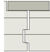
Variante 14 10 mm Nut und Feder Standardausfaltung 23/51 mm Dicke 90–360 mm Sonderausfaltung max. 61/59 mm Dicke abhängig der Falztiefe
