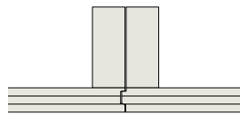
Variante 41 10 mm Nut und Feder
