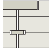
Variante 15 9 x 30 mm Fremdfeder Standardausfaltung 23/51 mm alternativ 28/51 mm Dicke: 100–280 mm
