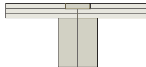
Variante 43 Standardausfaltung 23/51 mm alternativ 28/51 mm Gesamthöhe: 160–490 mm
