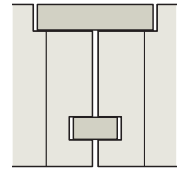
Variante 5 19 x 38 mm Fremdfeder Standardausfaltung 23/51 mm alternativ 28/51 mm
