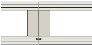
Variante 32 9 x 30 mm Fremdfeder CLT BOX – DECKE, Höhe: 220–480 mm CLT BOX – DECKE FS, Höhe: 260–490 mm
