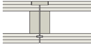
Variante 35 9 x 30 mm Fremdfeder Standardausfaltung 23/51 mm alternativ 28/51 mm CLT BOX – DECKE, Höhe: 220–480 mm CLT BOX – DECKE FS, Höhe: 260–490 mm
