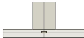
Variante 42 9 x 30 mm Fremdfeder Gesamthöhe: 160–490 mm
