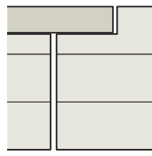
Variante 13 Standardausfaltung 23/51 mm alternativ 28/51 mm Dicke: 60–280 mm
