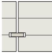
Variante 12 9 x 30 mm Fremdfeder Dicke: 60–280 mm
