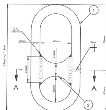
Bild 9: Abmessungen im Einhängebereich des Kugelkopfanfers
